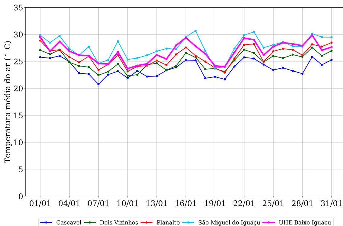
Figura 1: Temperatura média do ar observada na região da UHE Baixo Iguaçu em janeiro de 2019.
