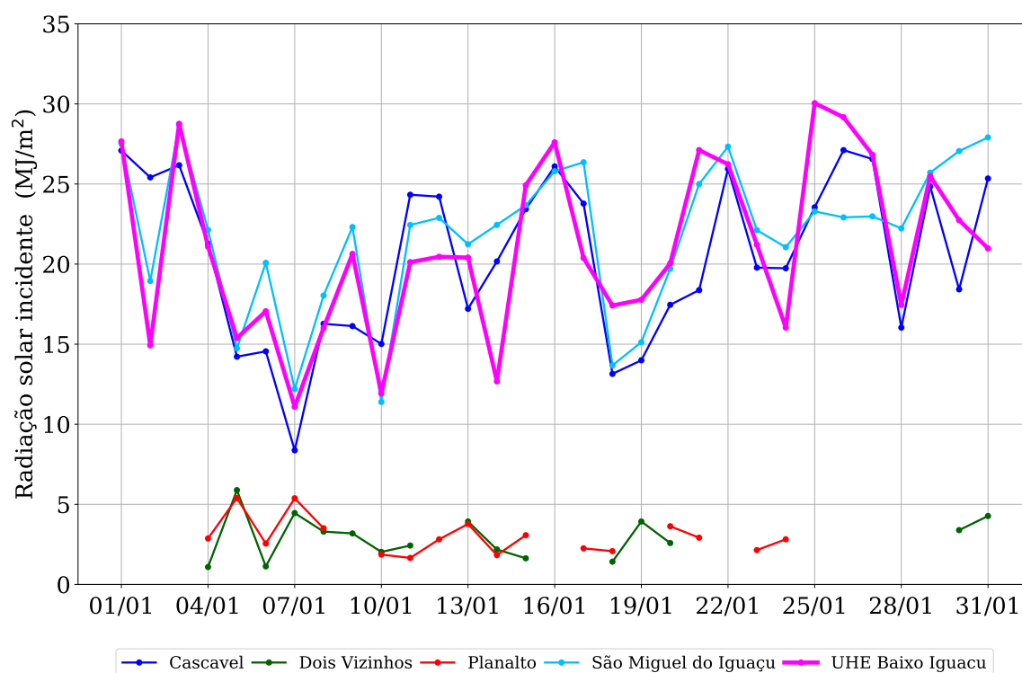
Figura 6: Radiação solar incidente observada na região da UHE Baixo Iguaçu em janeiro de 2019.
