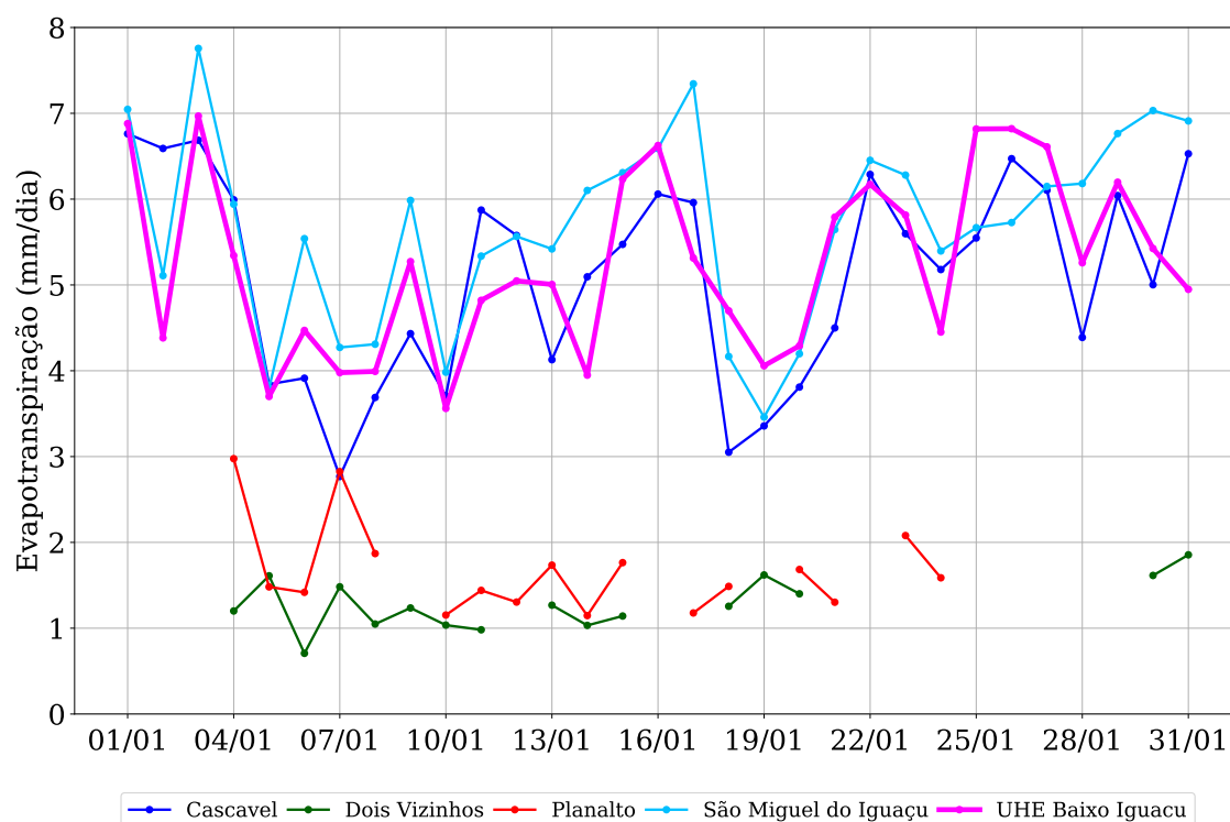
Figura 7: Evapotranspiração observada na região da UHE Baixo Iguaçu em janeiro de 2019.
