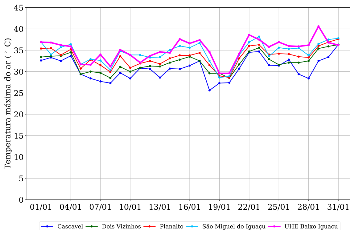
Figura 2: Temperatura máxima do ar observada na região da UHE Baixo Iguaçu em janeiro de 2019.
