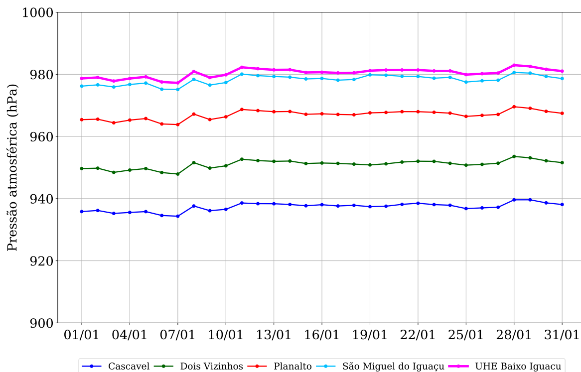
Figura 5: Pressão atmosférica observada na região da UHE Baixo Iguaçu em janeiro de 2019.
