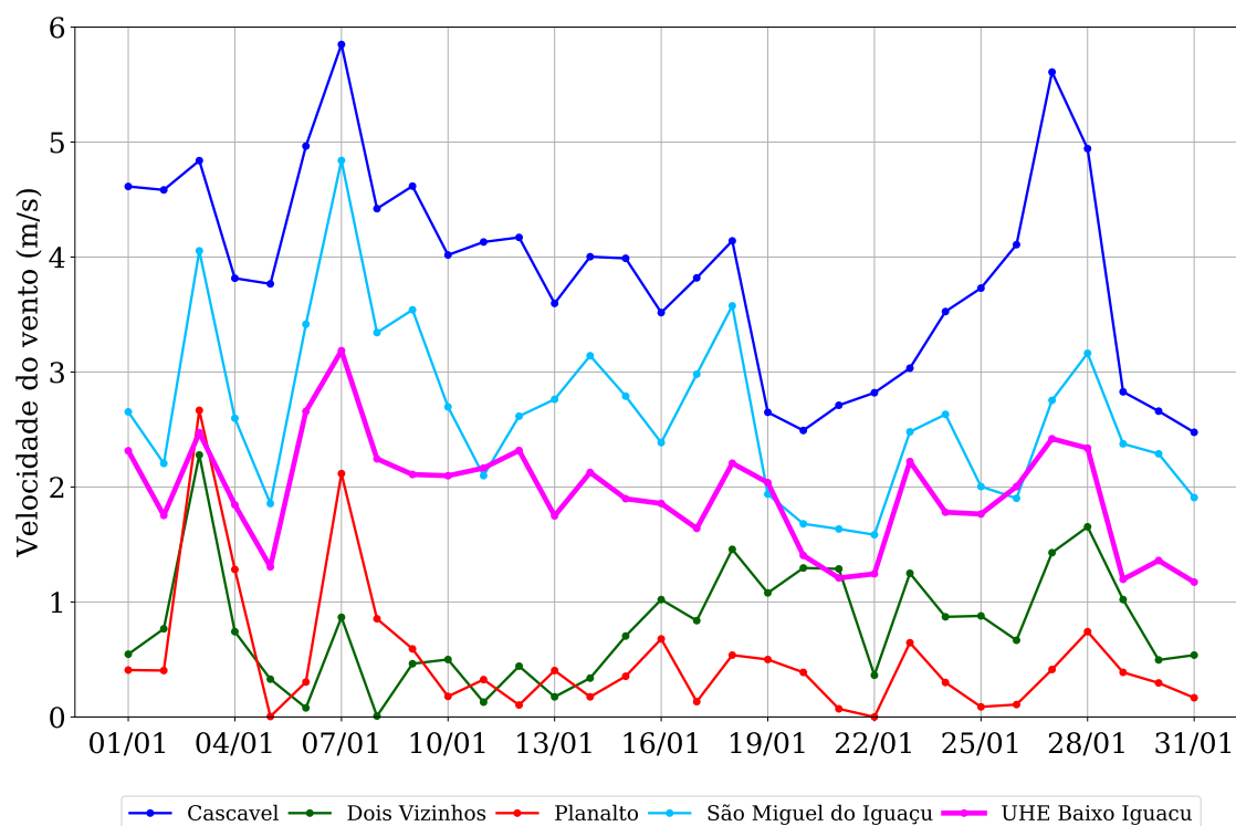
Figura 8: Velocidade observada na região da UHE Baixo Iguaçu em janeiro de 2019.
