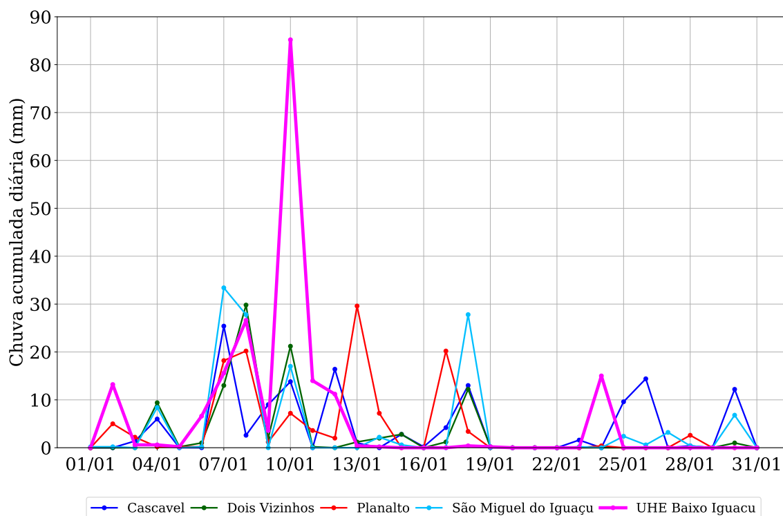
Figura 10: Registros de chuva acumulada diária observada na região da UHE Baixo Iguaçu ao longo de janeiro de 2019.
