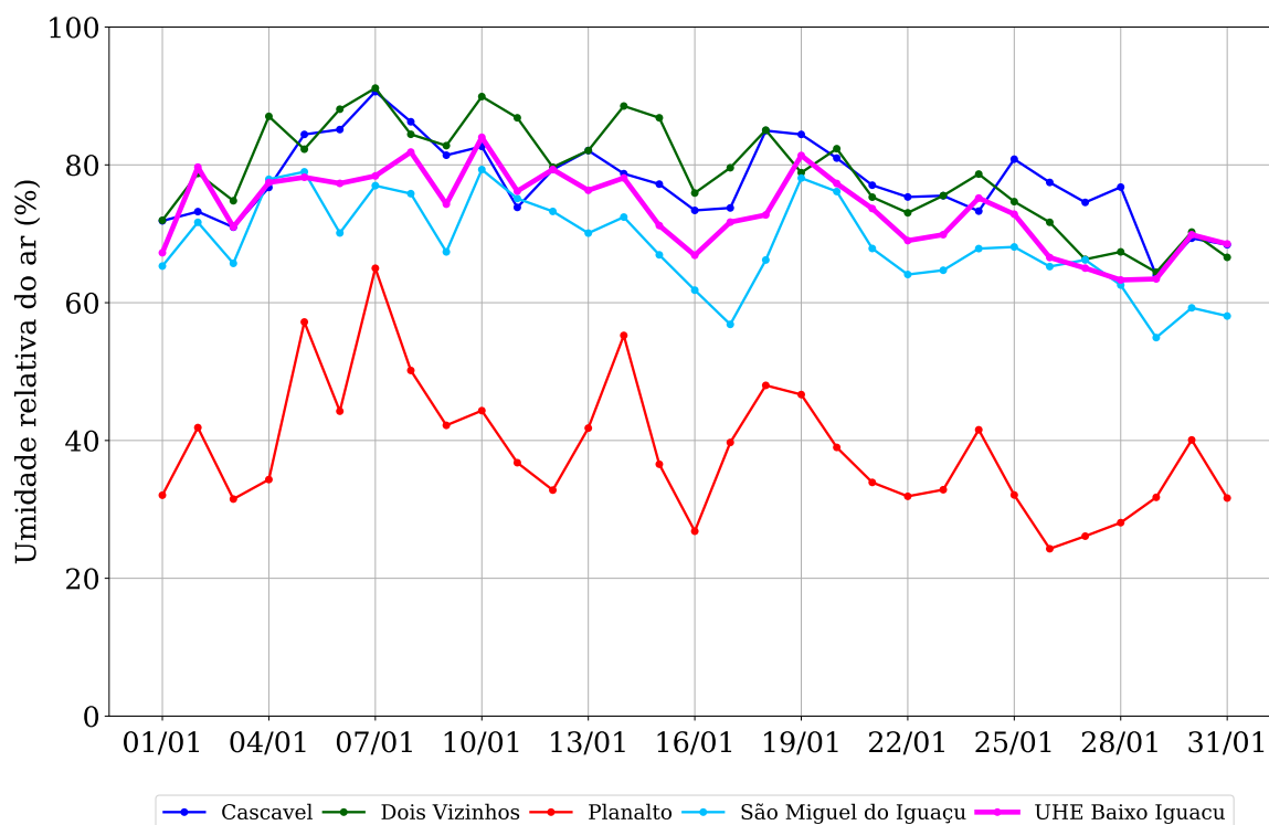
Figura 4: Umidade relativa observada na região da UHE Baixo Iguaçu em janeiro de 2019.
