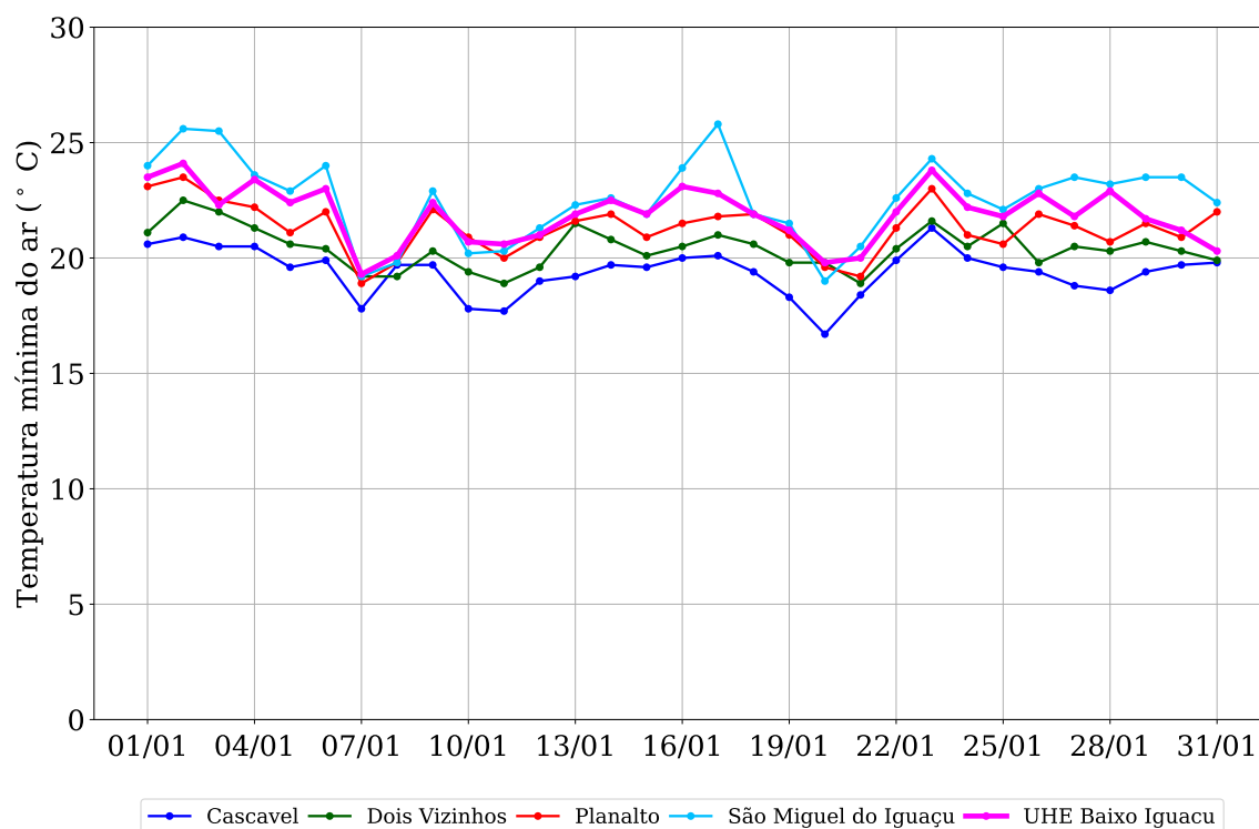
Figura 3: Temperatura mínima do ar observada na região da UHE Baixo Iguaçu em janeiro de 2019.
