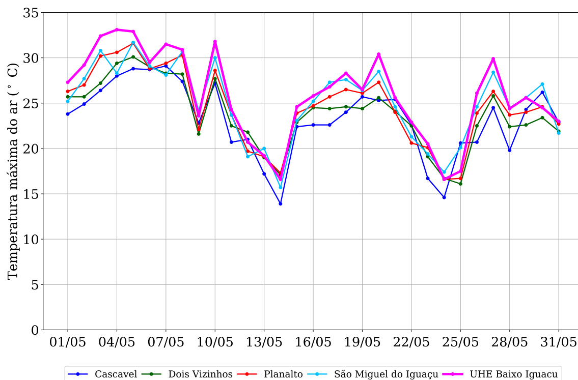
Figura 2: Temperatura máxima do ar observada na região da UHE Baixo Iguaçu em maio de 2019.
