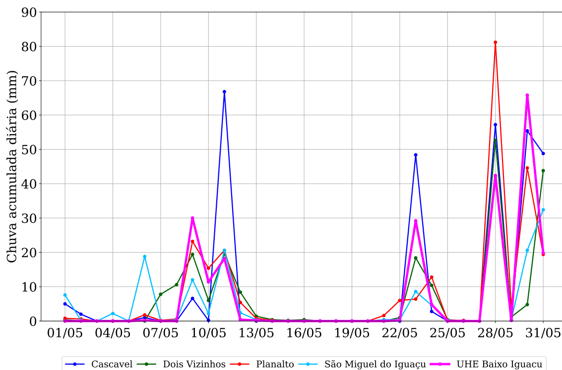
Figura 10: Registros de chuva acumulada diária observada na região da UHE Baixo Iguaçu ao longo de maio de 2019.
