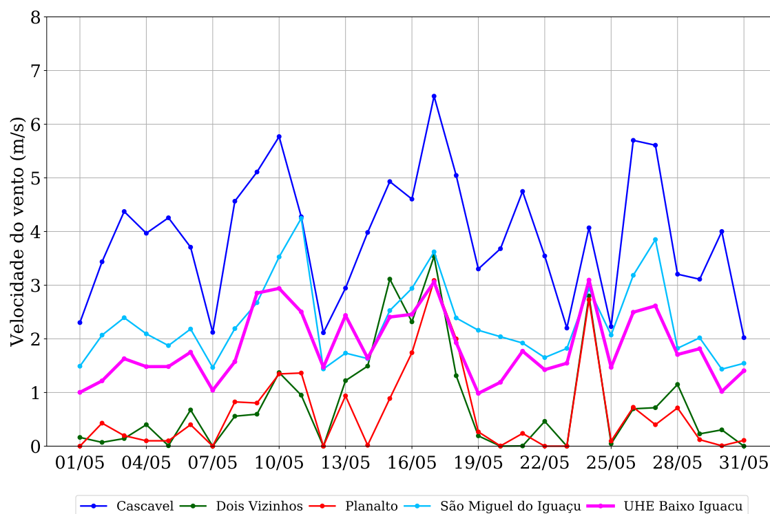
Figura 8: Velocidade observada na região da UHE Baixo Iguaçu em maio de 2019.
