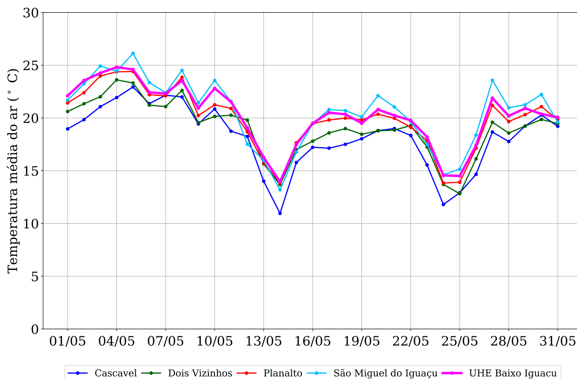
Figura 1: Temperatura média do ar observada na região da UHE Baixo Iguaçu em maio de 2019.
