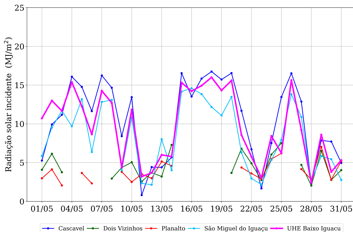
Figura 6: Radiação solar incidente observada na região da UHE Baixo Iguaçu em maio de 2019.
