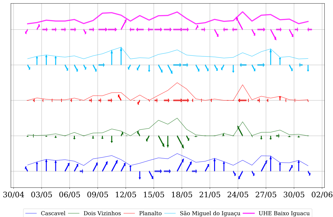
Figura 9: Diagrama da direção do vento predominante registrada nas estações meteorológicas na região da UHE Baixo Iguaçu.
