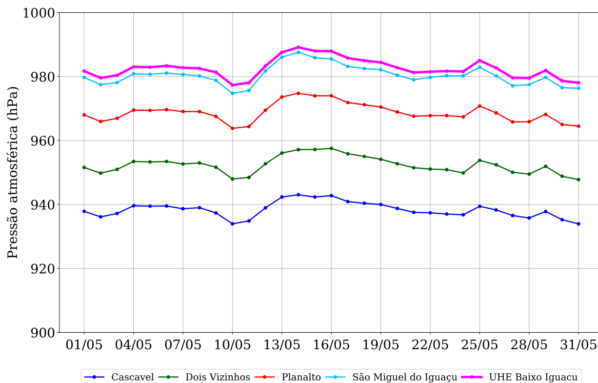
Figura 5: Pressão atmosférica observada na região da UHE Baixo Iguaçu em maio de 2019.
