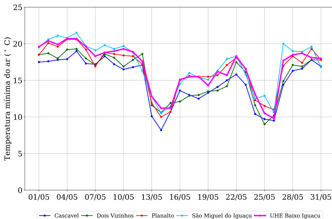
Figura 3: Temperatura mínima do ar observada na região da UHE Baixo Iguaçu em maio de 2019.
