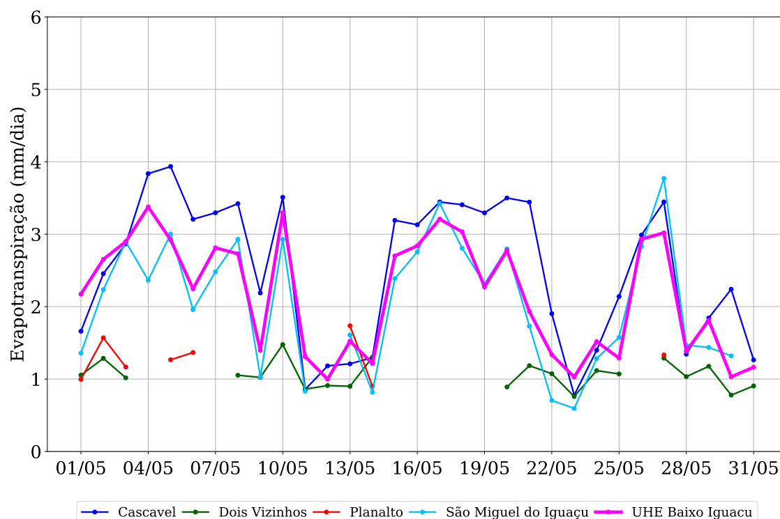
Figura 7: Evapotranspiração observada na região da UHE Baixo Iguaçu em maio de 2019.
