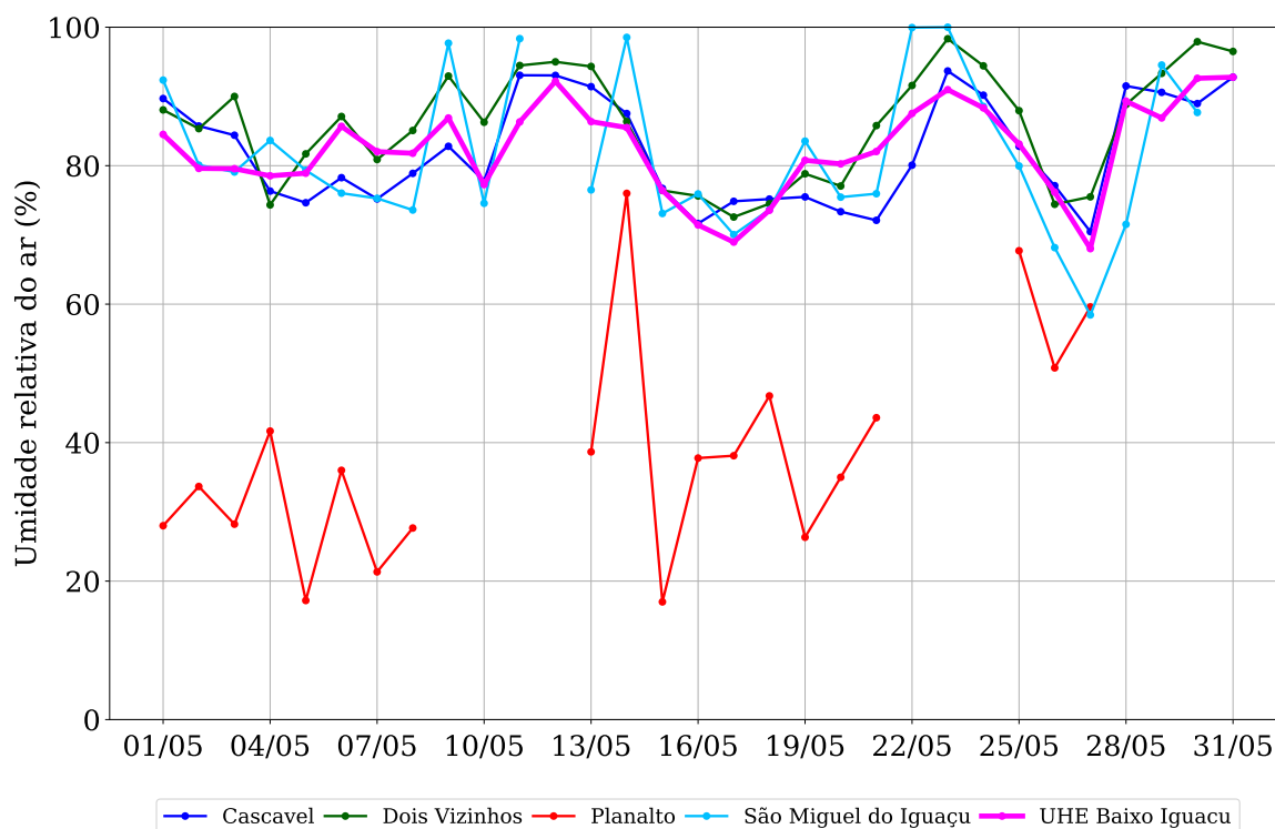
Figura 4: Umidade relativa observada na região da UHE Baixo Iguaçu em maio de 2019.
