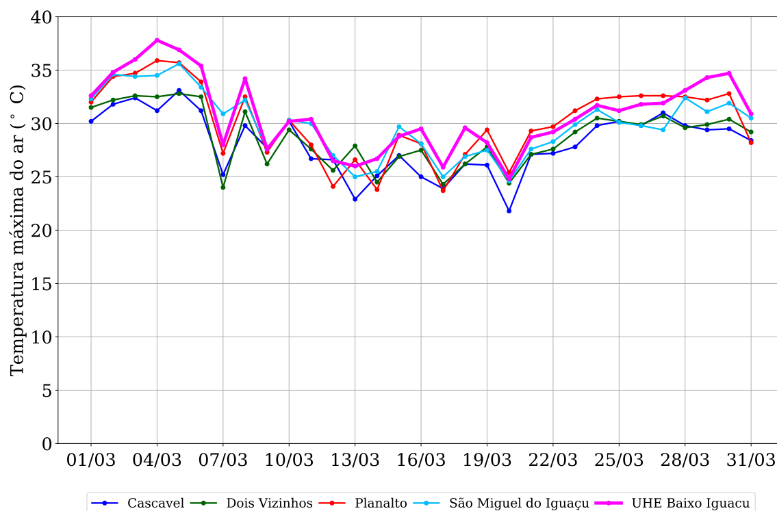
Figura 2: Temperatura máxima do ar observada na região da UHE Baixo Iguaçu em março de 2019.
