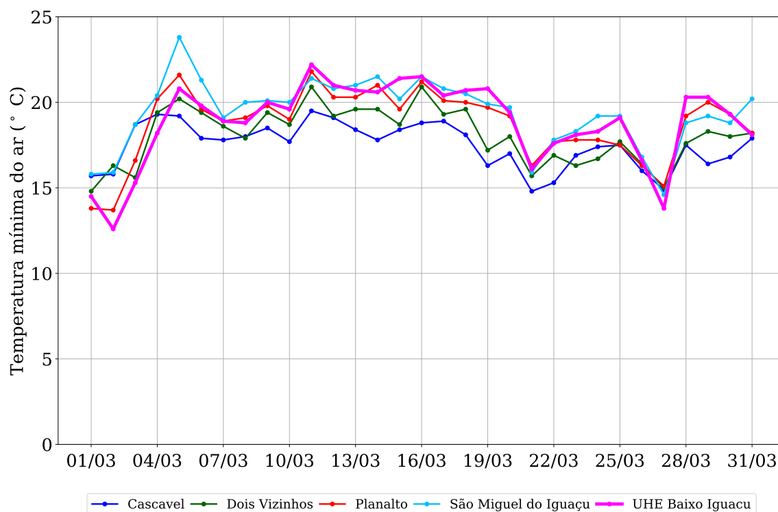
Figura 3: Temperatura mínima do ar observada na região da UHE Baixo Iguaçu em março de 2019.
