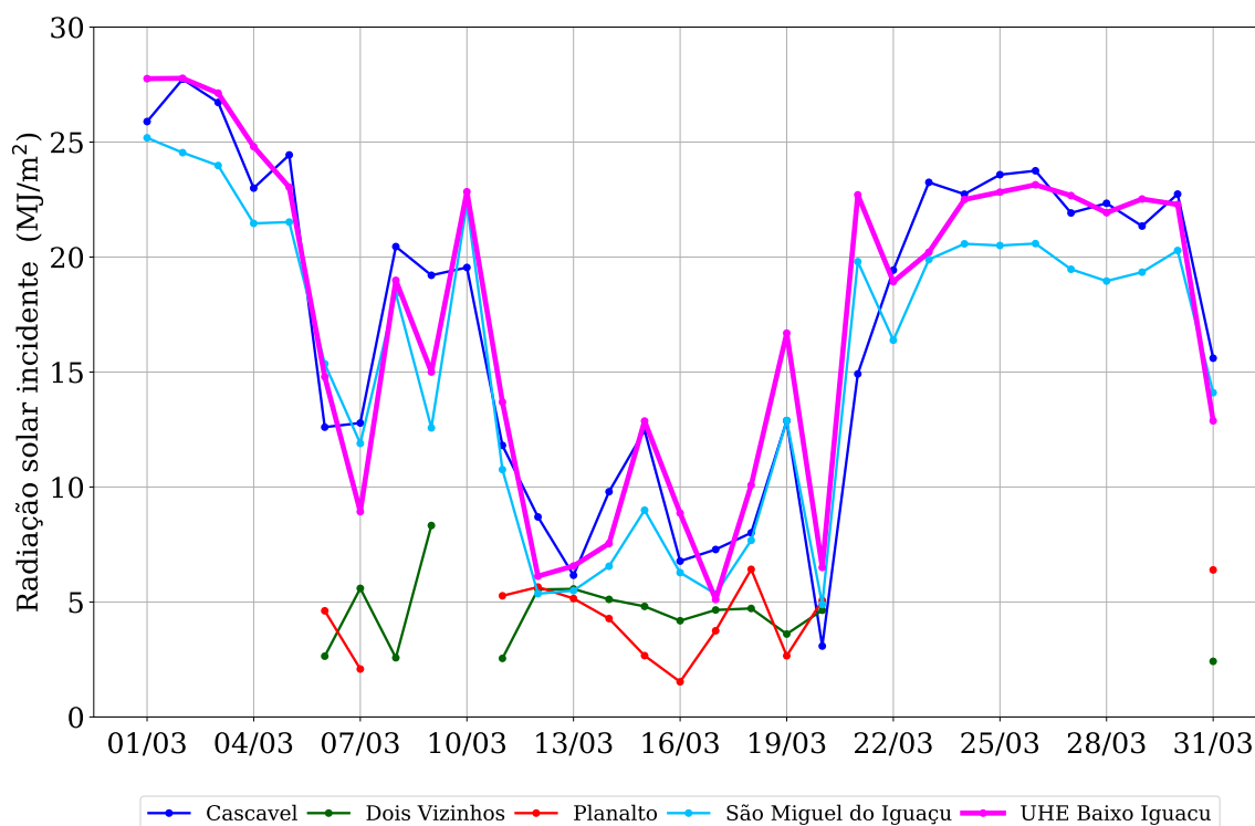
Figura 6: Radiação solar incidente observada na região da UHE Baixo Iguaçu em março de 2019.
