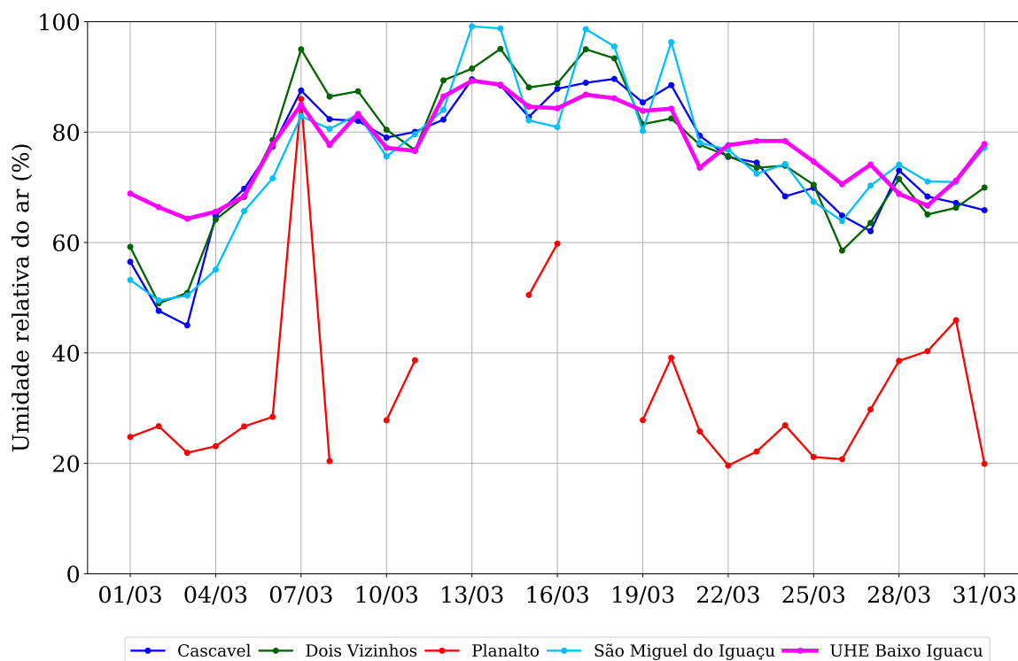
Figura 4: Umidade relativa observada na região da UHE Baixo Iguaçu em março de 2019.
