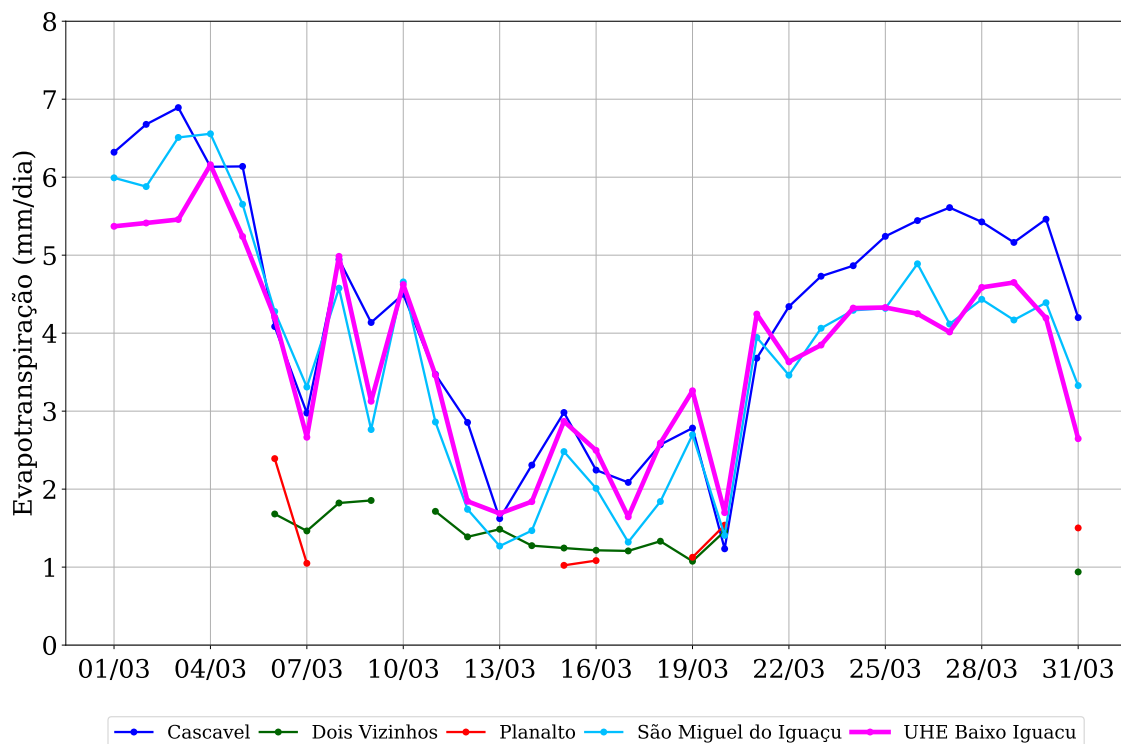
Figura 7: Evapotranspiração observada na região da UHE Baixo Iguaçu em março de 2019.
