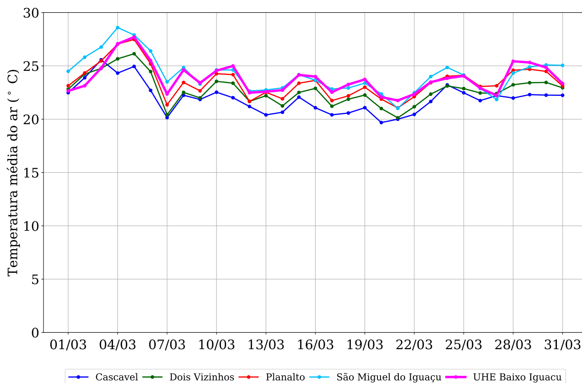
Figura 1: Temperatura média do ar observada na região da UHE Baixo Iguaçu em março de 2019.
