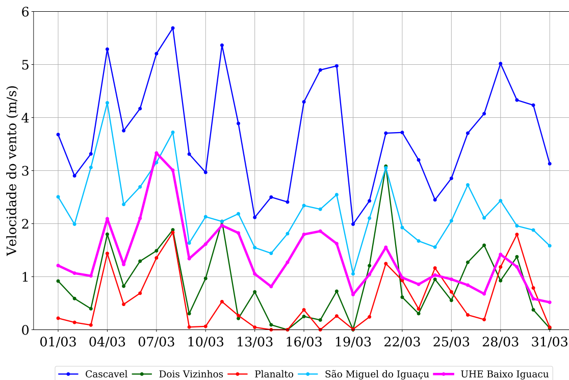
Figura 8: Velocidade observada na região da UHE Baixo Iguaçu em março de 2019.
