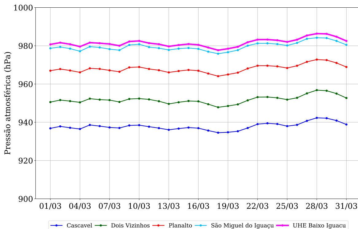
Figura 5: Pressão atmosférica observada na região da UHE Baixo Iguaçu em março de 2019.
