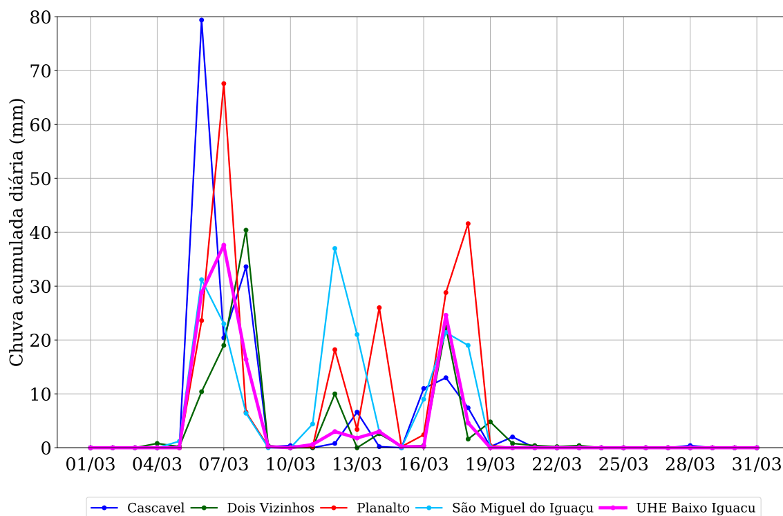
Figura 10: Registros de chuva acumulada diária observada na região da UHE Baixo Iguaçu ao longo de março de 2019.
